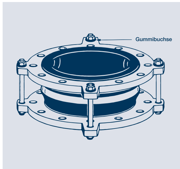
Standardausführung mit geräuschabsorbierenden Bewegungsbegrenzern
