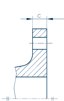
Form/Type A Glatte Dichtfläche
