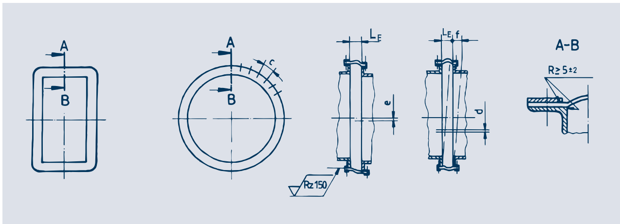
Band-Form Kompensator (z.B. Typ 120)
