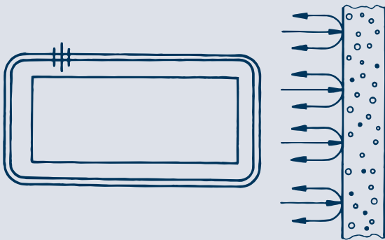
Nahtanordnung bei behinderter Wärmeabgabe durch eine Wand
