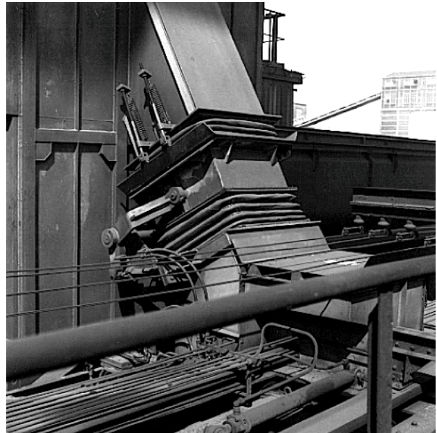
Kompensator am Haubenwagen einer Kokerei
