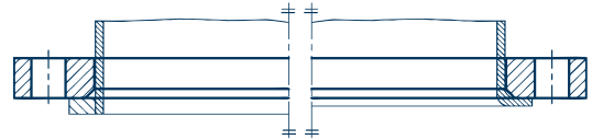
Typ 02 Loser Flansch für glatten Bund Typ 32, oder für gebördeltes Rohrende, Typ 33
