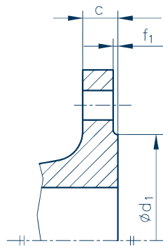
Form/Type B Dichtleiste (B1 und B2)*
