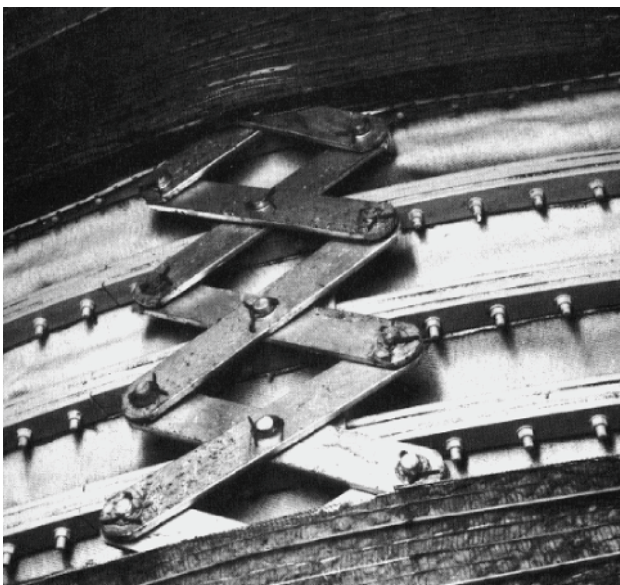
Kompensator im Kamin eines Kohlekraftwerks
