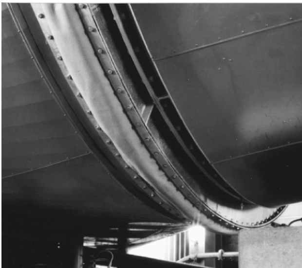
Kempchen-Kompensator in einer Rauchgas-Sammelleitung.
