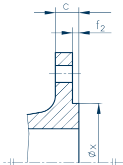
Form/Type E Vorsprung
