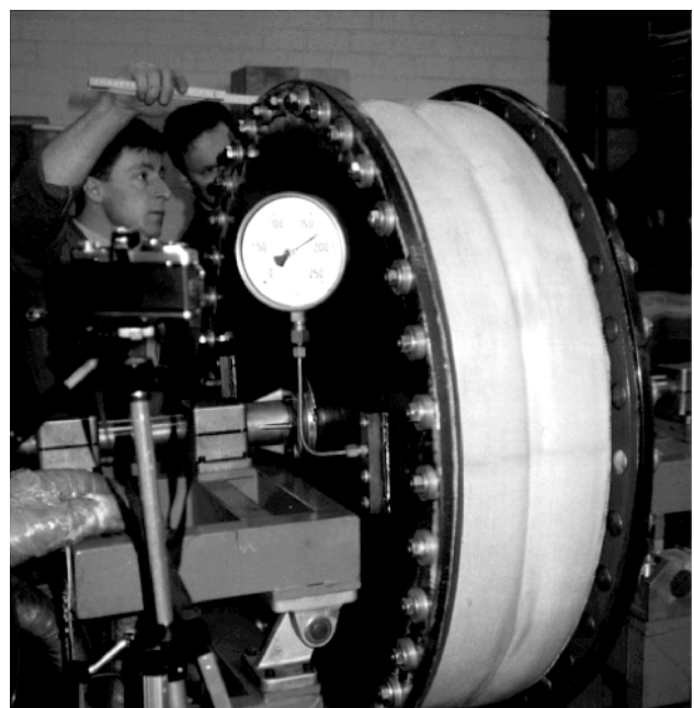
Mitarbeiter bei der Druckprüfung eines Kompensators am Kempchen-Kompensatorenprüfstand
