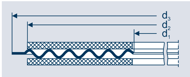
Profil: W1A-3
