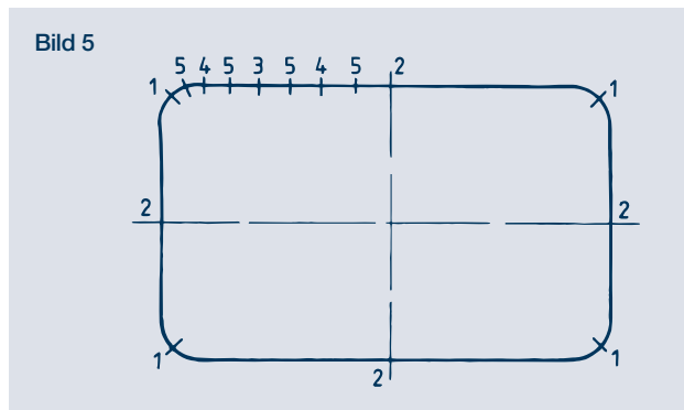
Verschraubungsschema für eckige Kompensatoren
