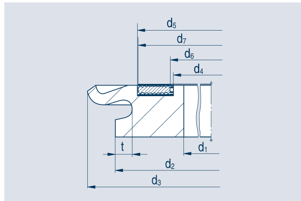
Profil A23N
