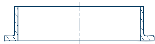
Typ 36 Pressbördel mit langem Ansatz
