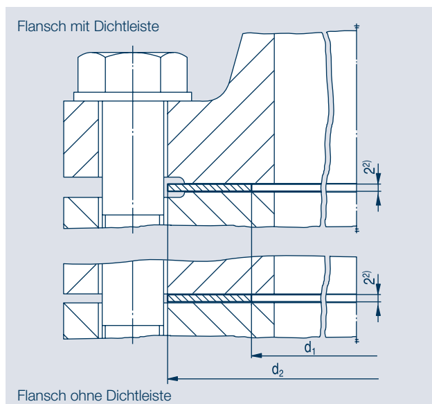
Nach EN 1514-1 Form IBC
