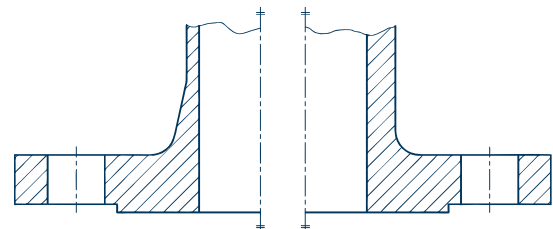
Typ 21 Integralflansch
