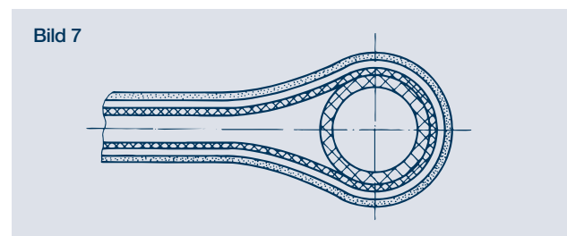
Knickschutz durch Papprollen
