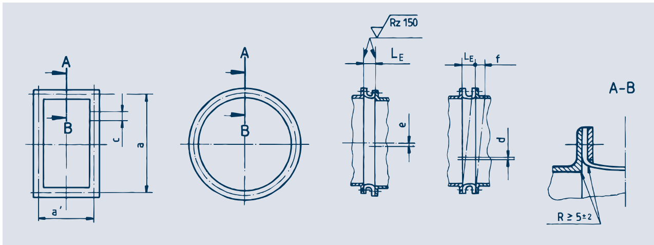
U-Form Kompensator (z.B. Typ 110)
