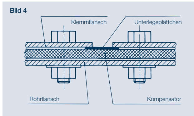
Anordnung der Unterlegeplättchen
