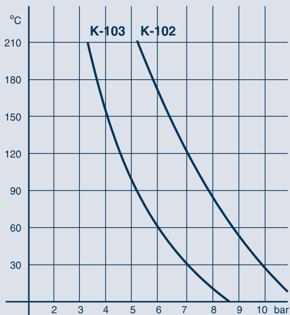
Temperatur-Betriebsdruck-Schaubild
