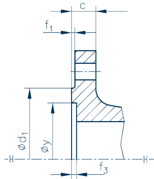
Form/Type F Rücksprung
