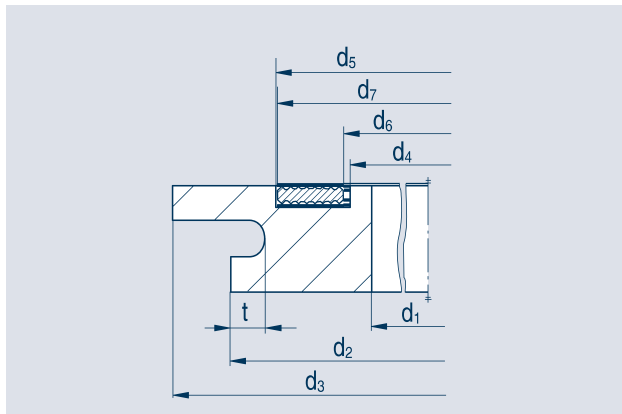
Profil A22N
