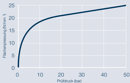
Gasdichtheitskurve
