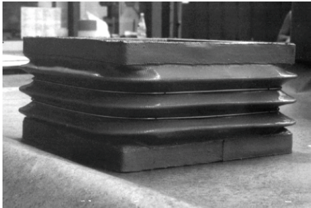
Rechteck-Faltenkompensator
