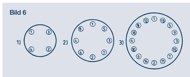
Verschraubungsschema für runde Kompensatoren
