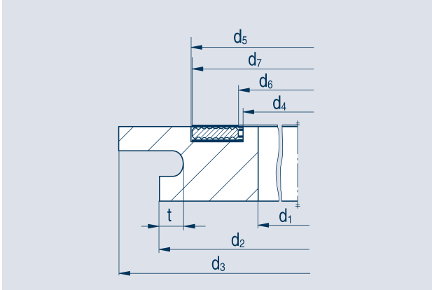
Profile A22N
