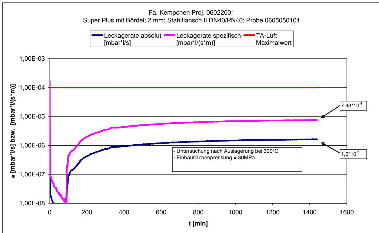
Probe 0605050101; Leckageuntersuchung bei 1 bar Prüfdruck
